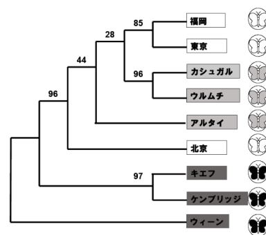
図 1. モンシロチョウの系統。個体群名は、黒が欧州、灰が中央アジア、白が東アジア。雌の紫外線反射は欧州が弱く、東アジアは強い。中央アジアは中間的。各分岐の上の数字はブートストラップ値。
