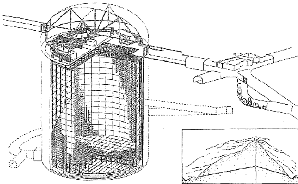
【図2】スーパーカミオカンデの概要
