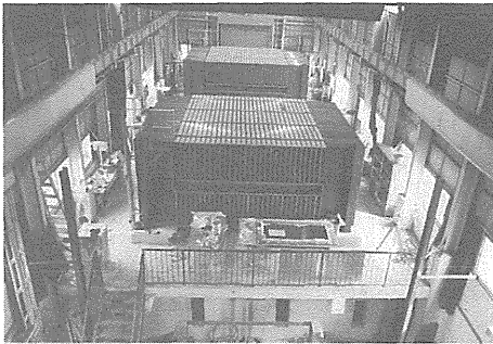
【写真1】ミュートロン(宇宙線ミュオン測定用電磁石スペクトロメータ)
