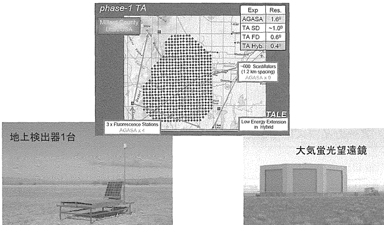
【図3】望遠鏡アレイ(TA)実験
